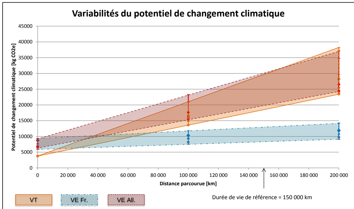
Figure 1-6 : Variabilités du potentiel de changement climatique pour les véhicules électriques français et allemand et les véhicules thermiques essence et diesel en 2012
